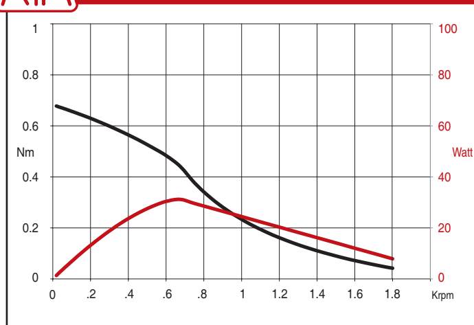
SANYO 103 H7123 5040 Collegamento bipolare 24 V 2 Amp
