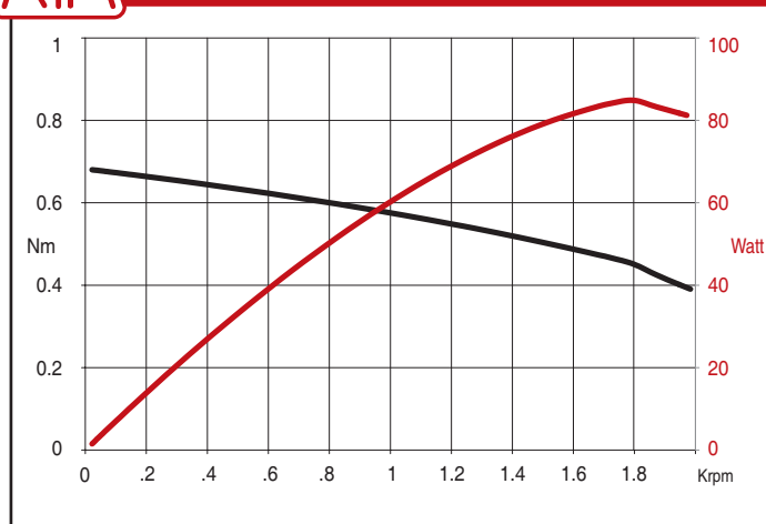
SANYO 103 H7123 5040 Collegamento bipolare 65 V 2 Amp
