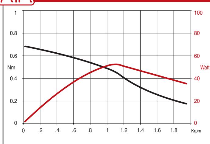
SANYO 103 H7123 5040 Collegamento bipolare 40 V 2 Amp
